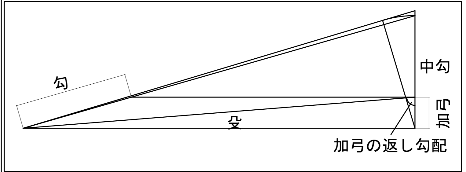
柱脚の癖 加弓勾配
